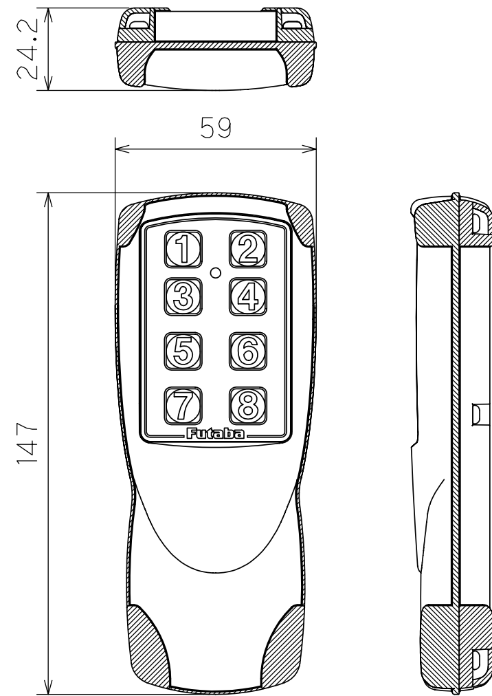
送信機
