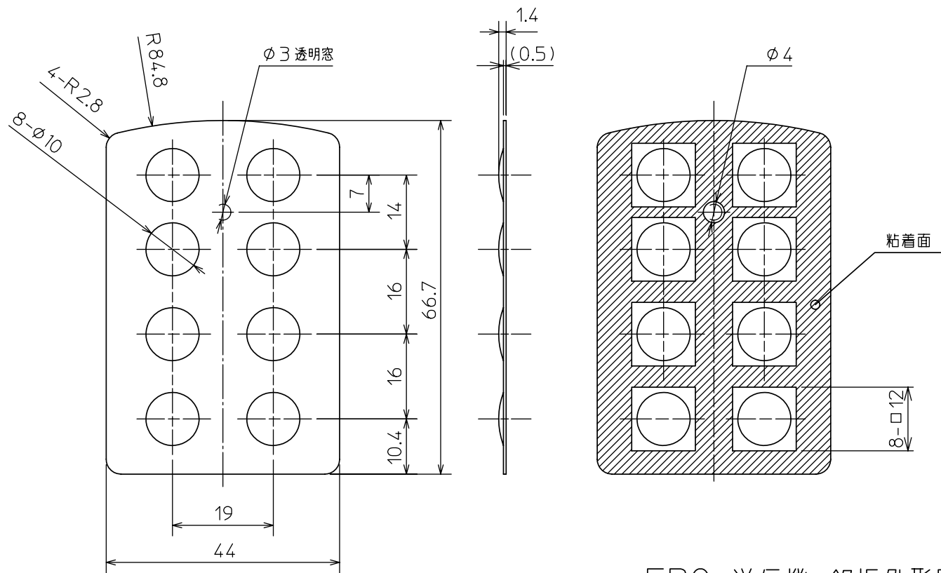
FRQ 送信機 銘板外形図
